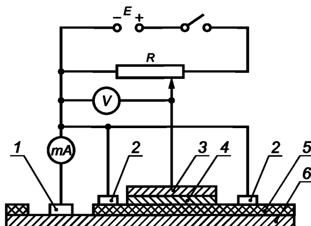
1 — контакт с трубой; 2 — экранирующие кольцевые электроды-бандаж; 3 — кольцевой электрод-бандаж; 4 — тканевое полотенце; 5 — защитное покрытие трубы; 6 — стенка трубы; E — источник постоянного тока; R — потенциометр; V — высокоомный вольтметр; mA — миллиамперметр
