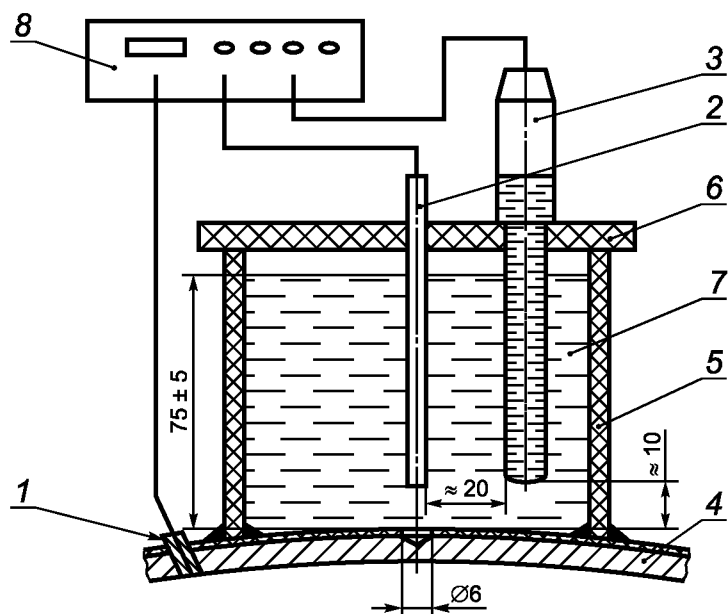
1 — катод; 2 — вспомогательный электрод (инертный анод); 3 — хлорсеребряный насыщенный электрод (электрод сравнения); 4 — карта или пластина с защитным покрытием (испытываемый образец); 5 — цилиндр; 6 — крышка; 7 — электролит; 8 — потенциостат
