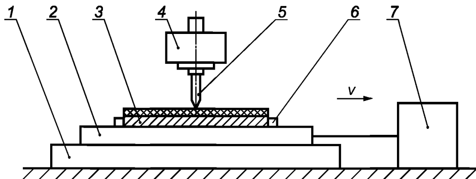
1 — основание; 2 — подвижная платформа; 3 — образец с покрытием; 4 — съемный груз; 5 — конусный резец; 6 — фиксаторы образца; 7 — регулируемый привод
